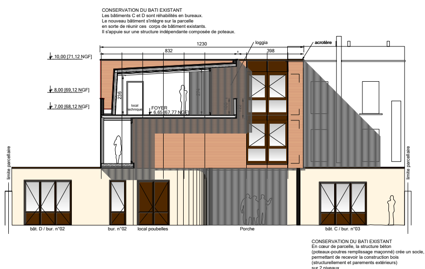
Elévation sur les bâtiments C et D
